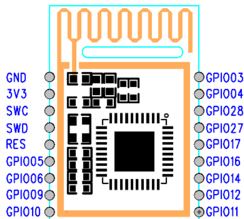
图 1-引脚定义
